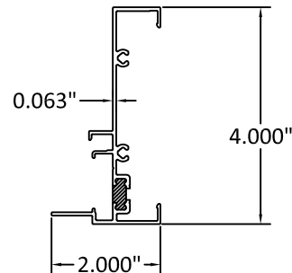
13 FRAME JAMB 6063-T5
