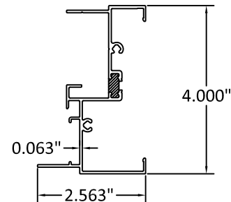
12 FRAME JAMB 6063-T5
